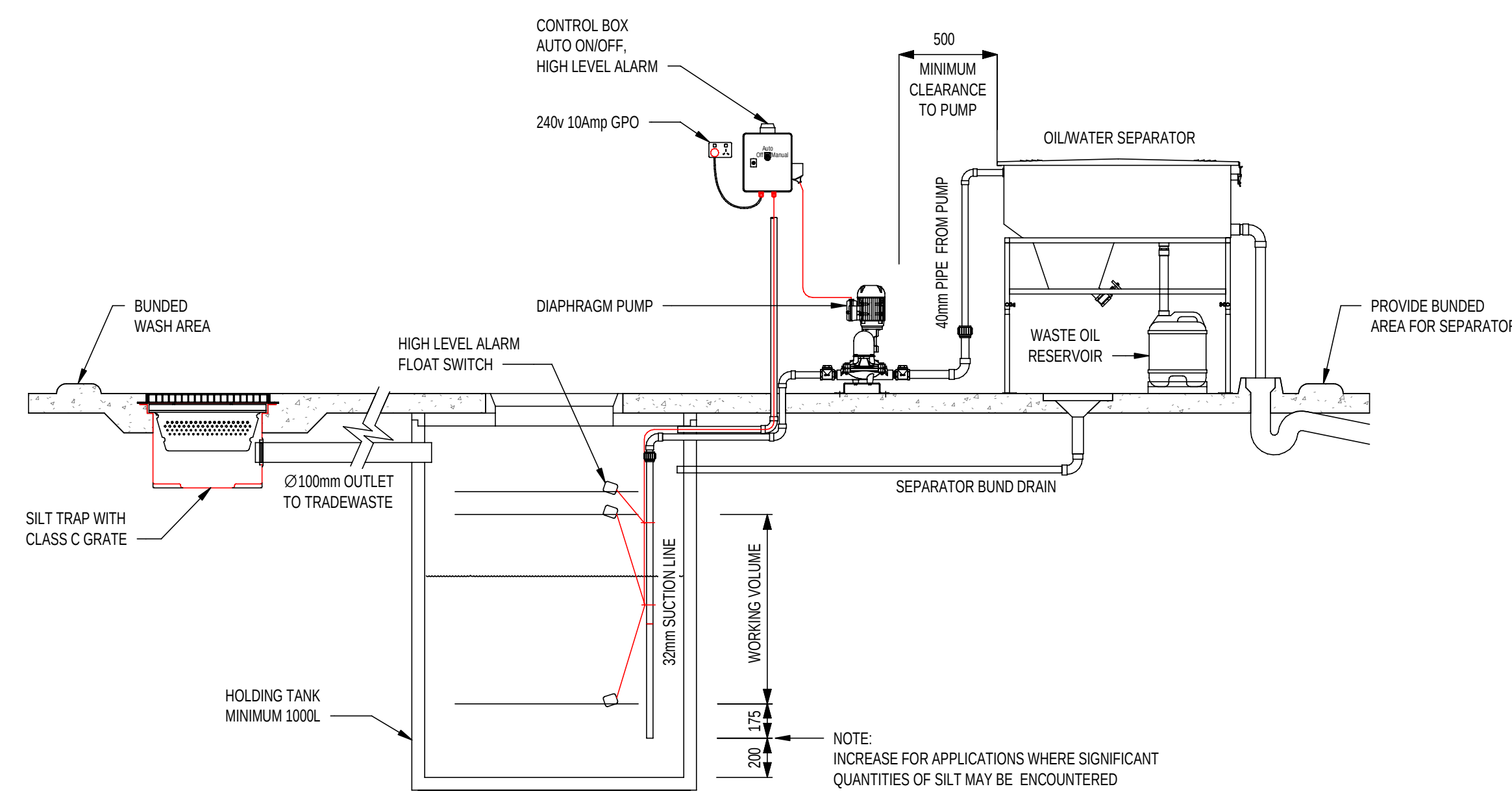
OIL/WATER SEPARATOR DETAIL N.T.S.
