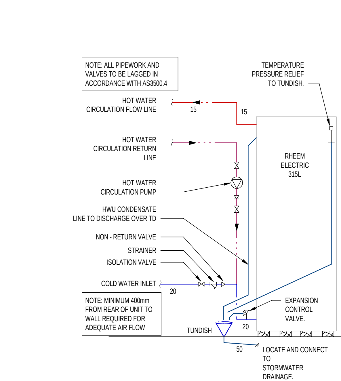
HOT WATER UNIT DETAIL N.T.S.
