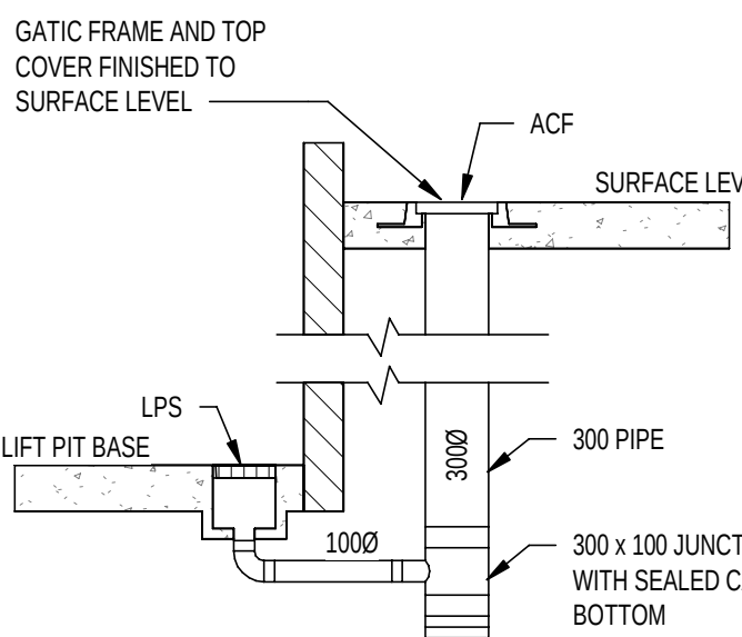
LIFT SUMP DRAINAGE N.T.S.
